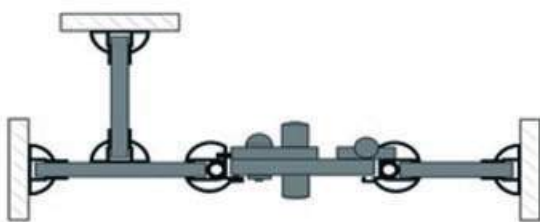
Schnittzeichnung VK 13 classic
