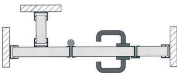
Schnittzeichnung SP 28 classic
