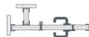
Schnittzeichnung SP 28 H
