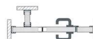
Schnittzeichnung SP 28 G
